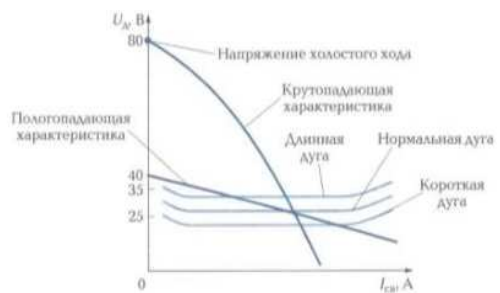
Рис. 1.6. Внешние характеристики источников питания и статическая вольт-амперная характеристика дуги
