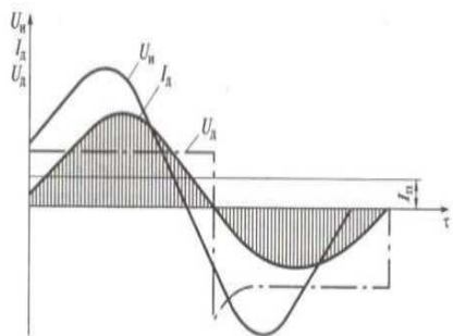
Рис. 2.5. Постоянная составляющая I_n силы тока в сварочной цепи при горении дуги на переменном токе: U_n — напряжение источника питания; U_d , I_d — напряжение и сила тока дуги; \tau — время
