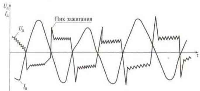
Рис. 2.4. Изменение полярности при горении дуги на переменном токе: U_d, I_d — напряжение и сила тока дуги
